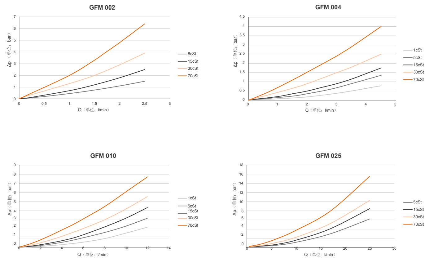
压力下降曲线
