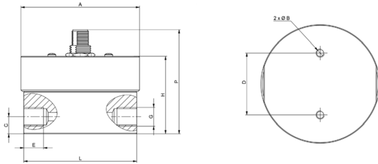
尺寸图
